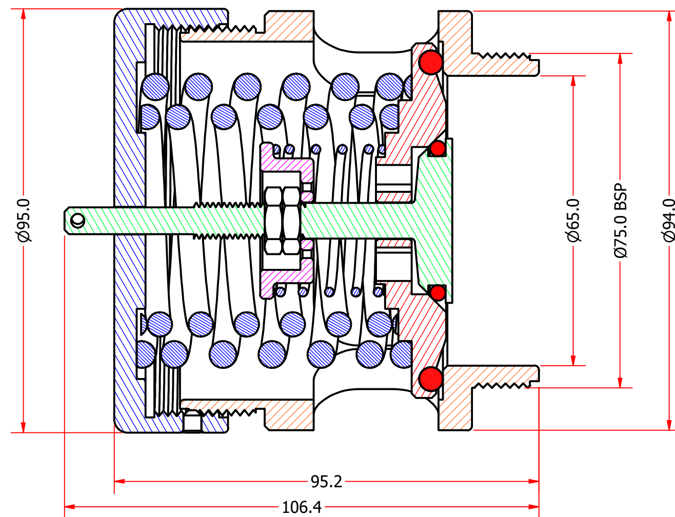
SECTION A-A SCALE 1.15 : 1
